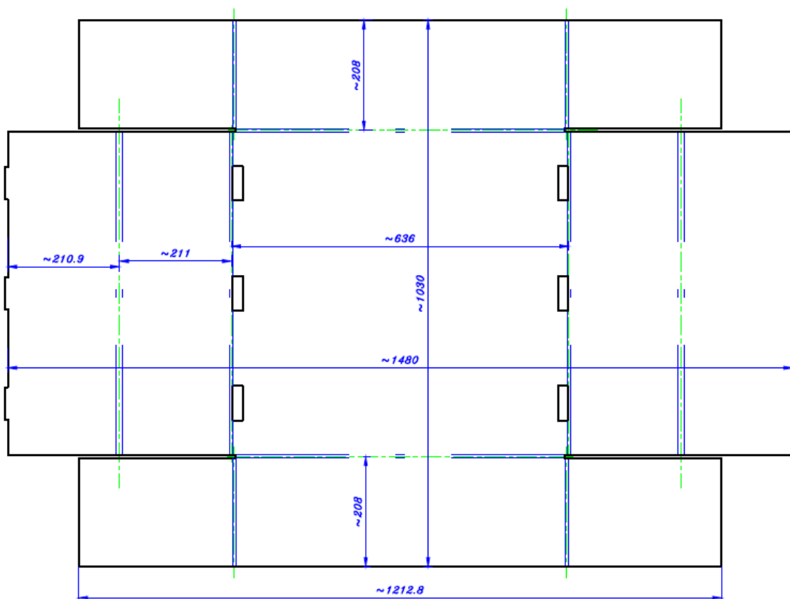
شماتیک کارتن دایکاتی در دو حالت بسته و گسترده
