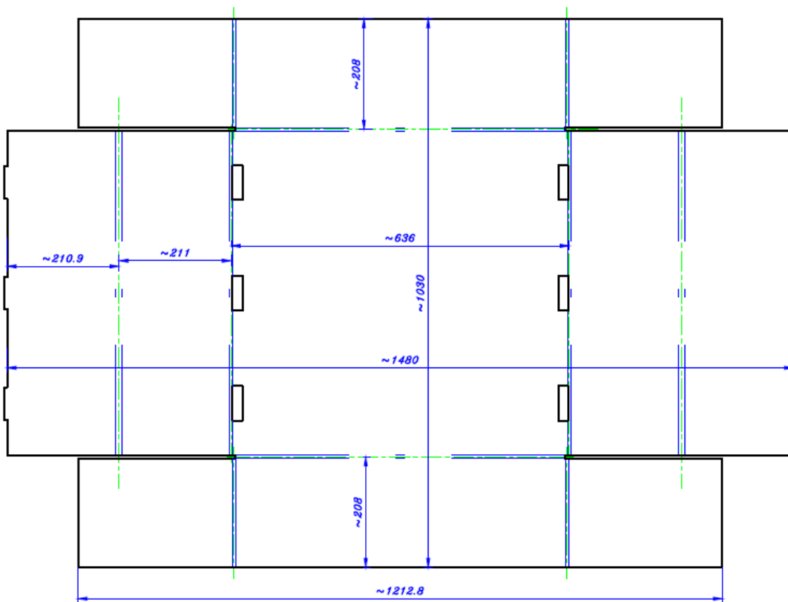
شماتیک کارتن دایکاتی در دو حالت بسته و گسترده
